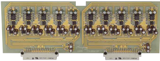
Diese Platine bildet die Lautstärkeregelung nach dem AAVA-Prinzip für einen Kanal
